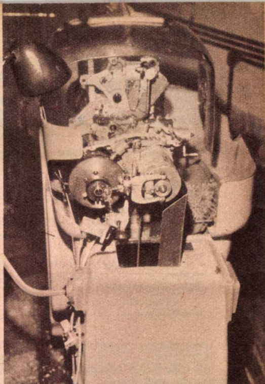
Munkában az üzem egyik legmodernebb gépe a AD-6/A típusú eszlelőszlovák gyártmányú esavarkészítő automata. Kapacitása: átlag 400 esavar óra
